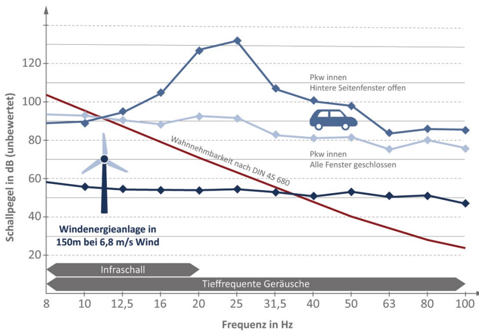
Abb. 1: Infrasschall und tieffrequente Geräusche von verschiedenen Emittenten
