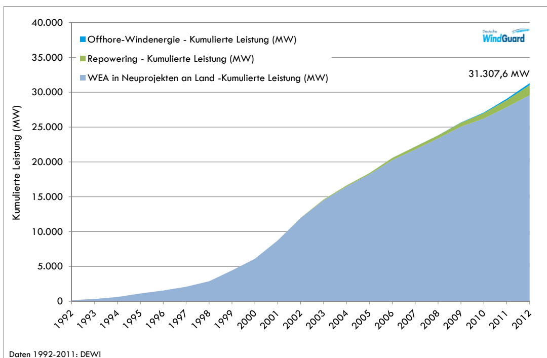
Abb. 2 Ausbauentwicklung der Windenergie in Deutschland – kumulierte Leistung (in MW), Status 31.12.2012
