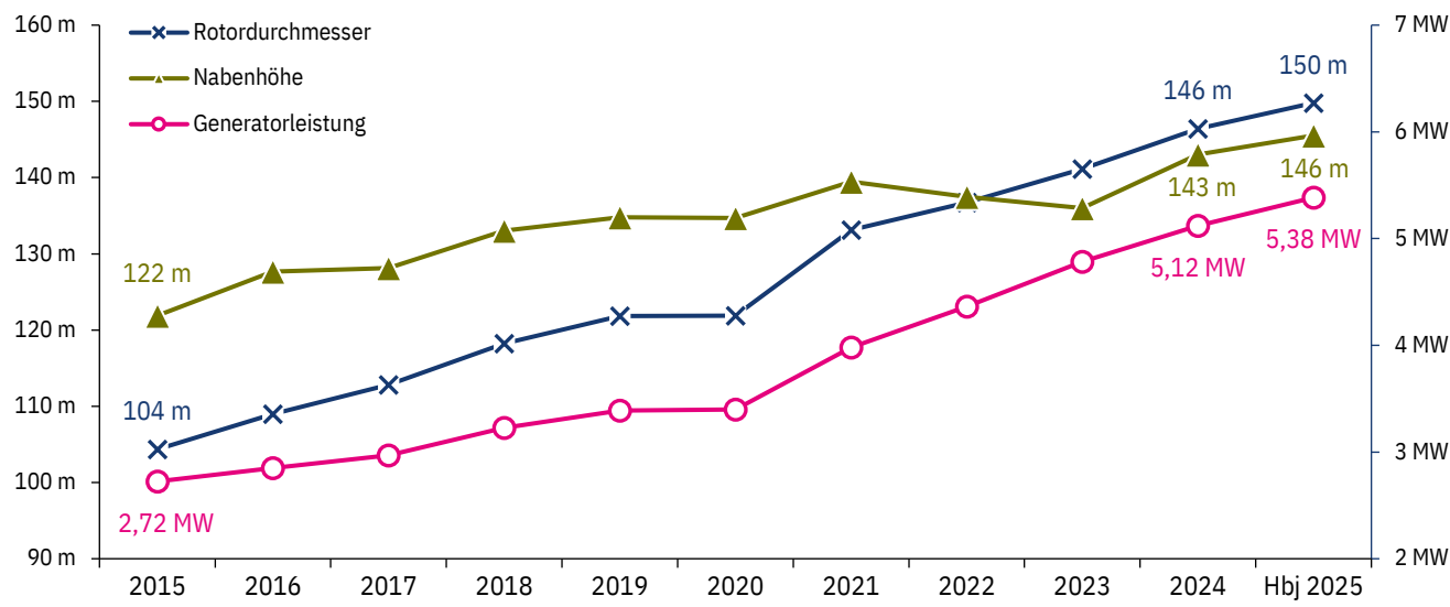
Abbildung 3: Durchschnittliche Konfiguration der jährlich in Betrieb gegangenen Windenergieanlagen
