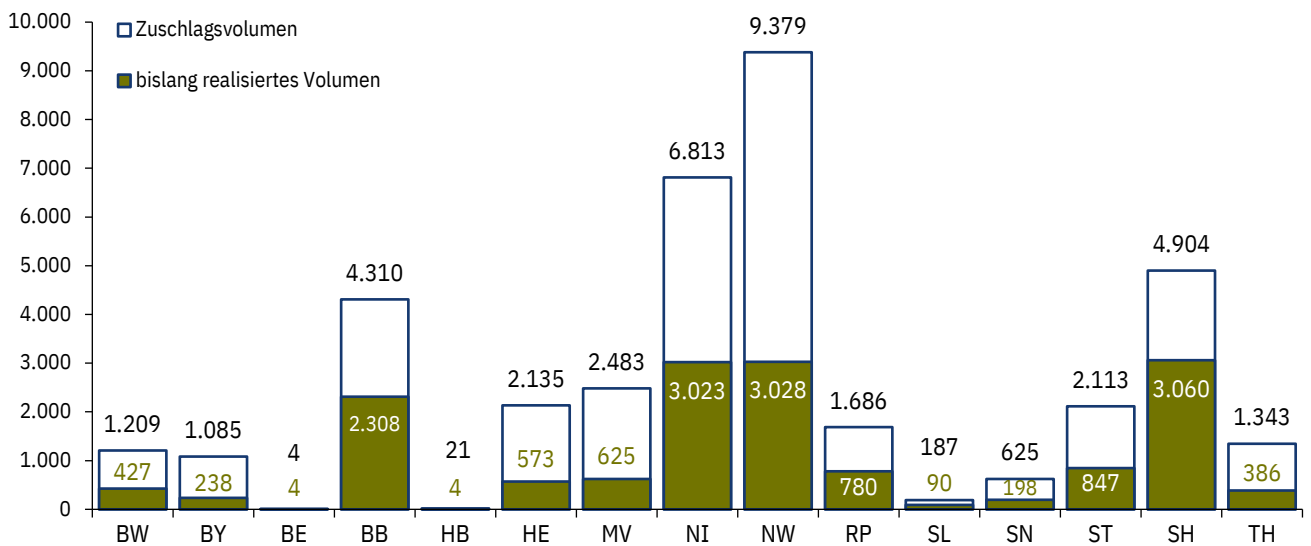
Abbildung 14: Bezuschlagte Windenergieleistung und bislang realisierte Anteile in den Ländern – ohne Ausschreibungsjahr 2017
