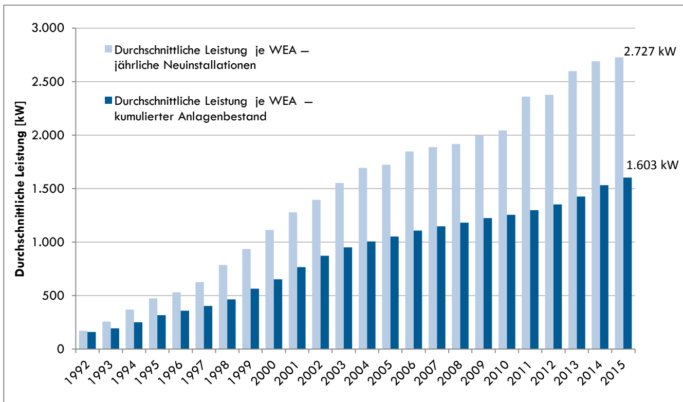
Abbildung 2: Entwicklung der durchschnittlichen Anlagenleistung der jährlich neu installierten WEA sowie der WEA im bundesweiten Gesamtbestand an Land, Status 31.12.2015
