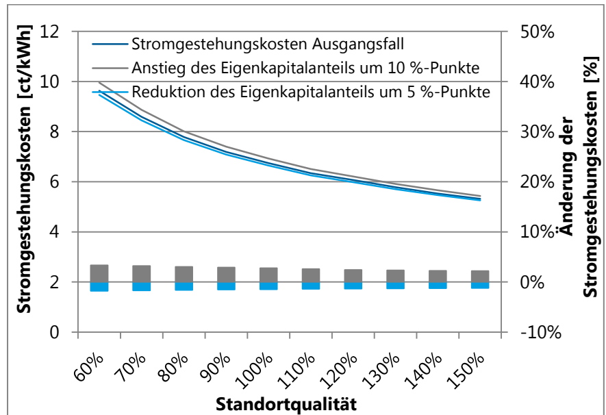
Abbildung 20: Auswirkung einer Veränderung des Eigenkapitalanteils auf die Stromgestehungskosten (ct/kWh) und prozentuale Veränderung. [eigene Berechnung]
