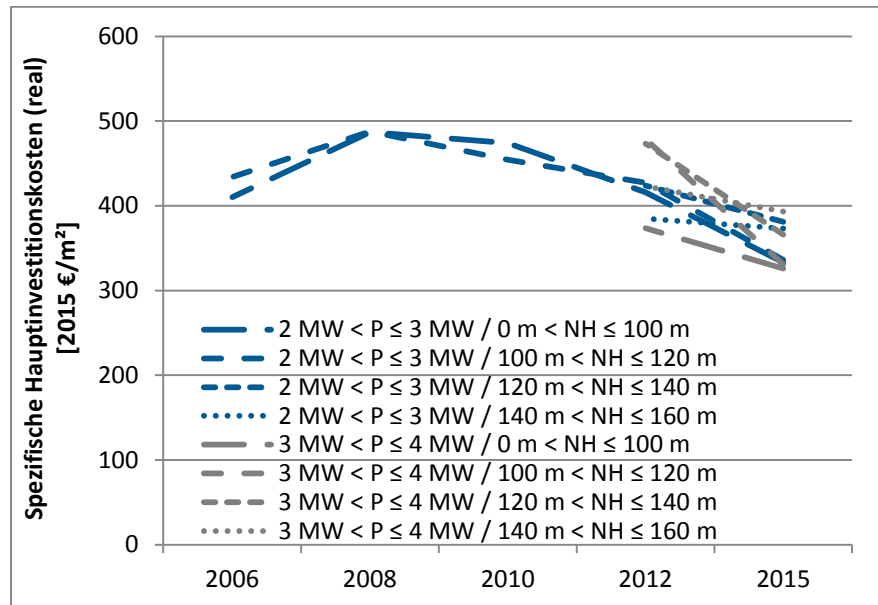
Abbildung 5: Zeitliche Entwicklung der spezifischen Haupt- investitionskosten pro Quadratmeter überstri- chener Rotorfläche von Windenergieanlagen der Leistungsklassen 2- 3 MW und 3-4 MW (in- flationsbereinigt) [DWG 2008, DWG 2011, DWG 2013]
