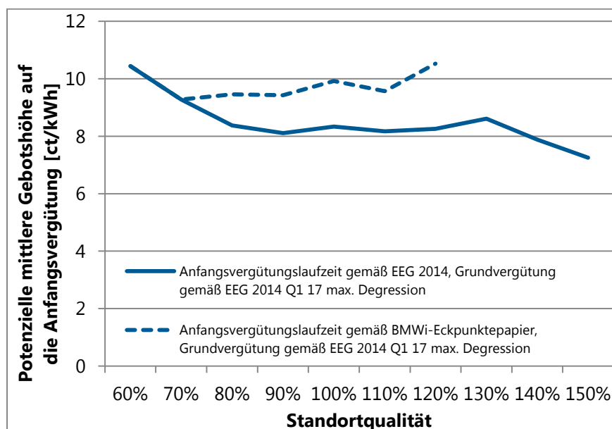
Abbildung 22: Potenzielle Gebotskurve im Ausschreibungssystem bei Gebot auf die Anfangsvergütung mit fixer Grundvergütungshöhe von 4,65 ct/kWh ( \triangleq Grundvergütung gemäß EEG 2014 im ersten Quartal 2017 bei maximaler Degression). Die Anfangsvergütungslaufzeiten werden gemäß EEG 2014 bzw. BMWi-Eckpunktepapier festgelegt.
