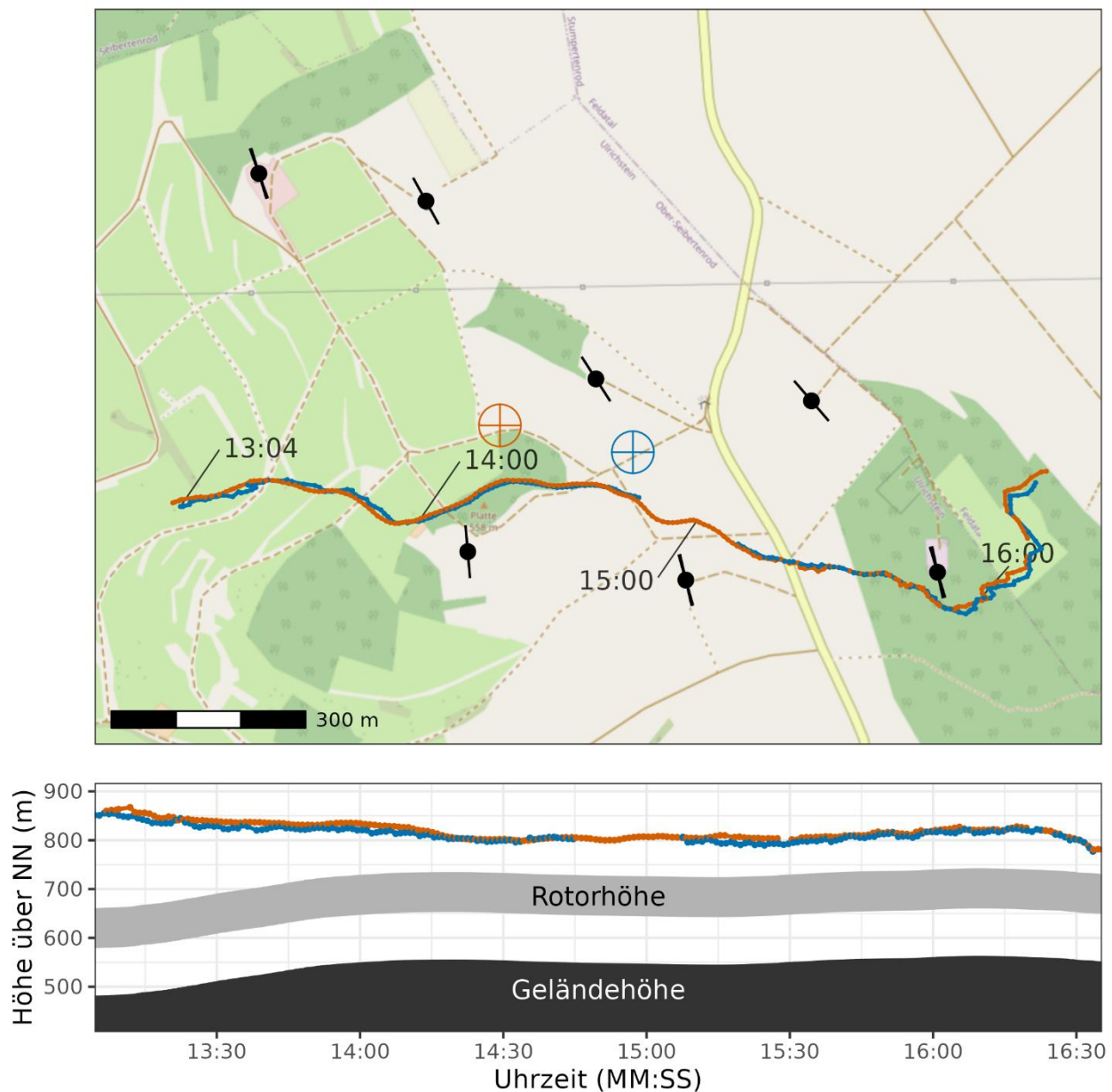
Abbildung 19: Dieselbe Beispielflughbahn nach der Rekalibrierung In der Kartendarstellung sind farblich kodiert die Messpunkte der 2 IDF-Systeme als Punkte eingetragen. Die Fadenkreuze stellen die jeweiligen Standorte der IDF-Systeme dar. Die WEA sind als schwarze Punkte eingezeichnet. Die zeitgleiche Rotorstellung(en) ist als schwarze Linien dargestellt. Die untere Grafik zeigt den Flughöhenverlauf der Rotmilanflughbahn. Die IDF-Messpunkte sind, gleich wie in der Karte, farblich unterschieden. Zusätzlich wird die Geländehöhe unter den jeweiligen Messpunkten als dunkelgrau unterlegte Fläche dargestellt. Aus der Geländehöhe abgeleitet wird darüber, hellgrau unterlegt, das Höhenband dargestellt, welches vom Rotor der WEA durchstreift wird.
