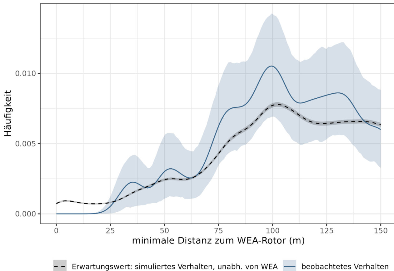
Abbildung 76: Häufigkeitsverteilung von pro Telemetrie-Flugbahn berechneten minimalen Annäherungsdistanzen von Rotmilanen an den WEA-Rotor. In der Darstellung wird die minimale Distanz zum Rotor verglichen zwischen aufgezeichneten Telemetrie-Flugbahnen (beobachtetes Verhalten) und simulierten Flugbahnen (Erwartungswert), die ein von den WEA unbeeinflusstes Flugverhalten darstellen sollen. Die Häufigkeitsverteilung, dargestellt als Linie, ist per Kerndichteschätzung (Gaußkern, h = 5 ) berechnet. Die schattierten Bereiche um die Linien stellen das 95 %-Sicherheitsintervall dar. Datengrundlage: 81 Flugbahnen, die zur Ermittlung des Erwartungswertes in 1 m Schritten, jeweils 0-200 m orthogonal zu ihrer Flugrichtung nach links und rechts verschoben wurden.
