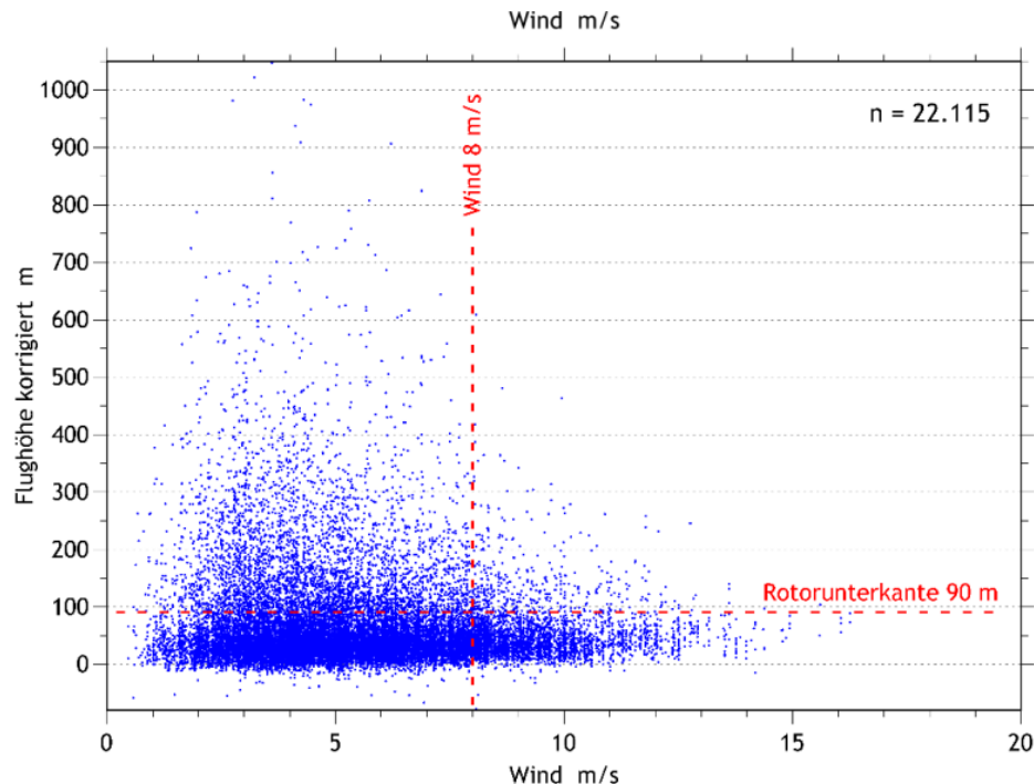
Abb. 5 a + b: Rotmilane im Flug als Flughöhe korrigiert (m) gegen Windgeschwindigkeit (m/s) im 5-Minuten-Datensatz im Anwesenheitszeitraum, nur Ortungspunkte im Flug. Daten der Besenderung von Juni 2016 bis Juli 2018. Datenquellen: Heuck et al. (2019), nachträglich ausgewertet vom HMWEVW. Zur Veranschaulichung wurde eine Windgeschwindigkeit von 8 m/s und eine Rotorunterkante von 80 m eingezeichnet
