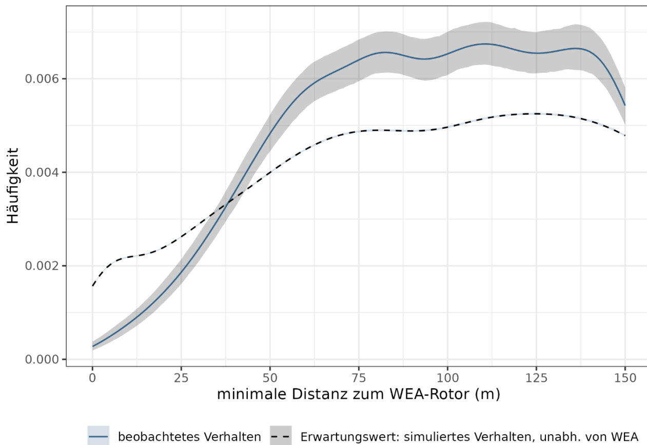
Abbildung 75: Häufigkeitsverteilung von pro IDF-Flugbahn berechneten minimalen Annäherungsdistanzen von Rotmilanen an den WEA-Rotor. In der Darstellung wird die minimale Distanz zum Rotor verglichen zwischen aufgezeichneten IDF-Flugbahnen (beobachtetes Verhalten) und simulierten Flugbahnen (Erwartungswert), die ein von den WEA unbeeinflusstes Flugverhalten darstellen sollen. Die Häufigkeitsverteilung, dargestellt als Linie, ist per Kerndichteschätzung (Gaußkern, h = 7,5 ) berechnet. Die schattierten Bereiche um die Linien stellen das 95 % Sicherheitsintervall dar. Datengrundlage: 2.034 Flugbahnen, die zur Ermittlung des Erwartungswertes in 1 m Schritten jeweils 0-200 m orthogonal zu ihrer Flugrichtung nach links und rechts verschoben wurden.
