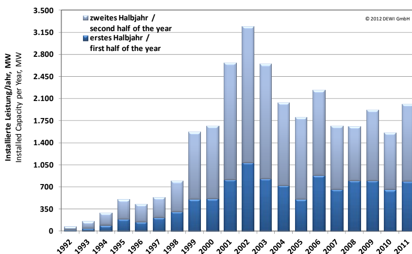
Abb. 1: Entwicklung der jährlichen installierten Leistung.
